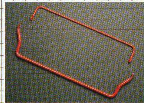
STABILISATEURS N001 V8 041F (avant) N001 V8 042F (arrière)
