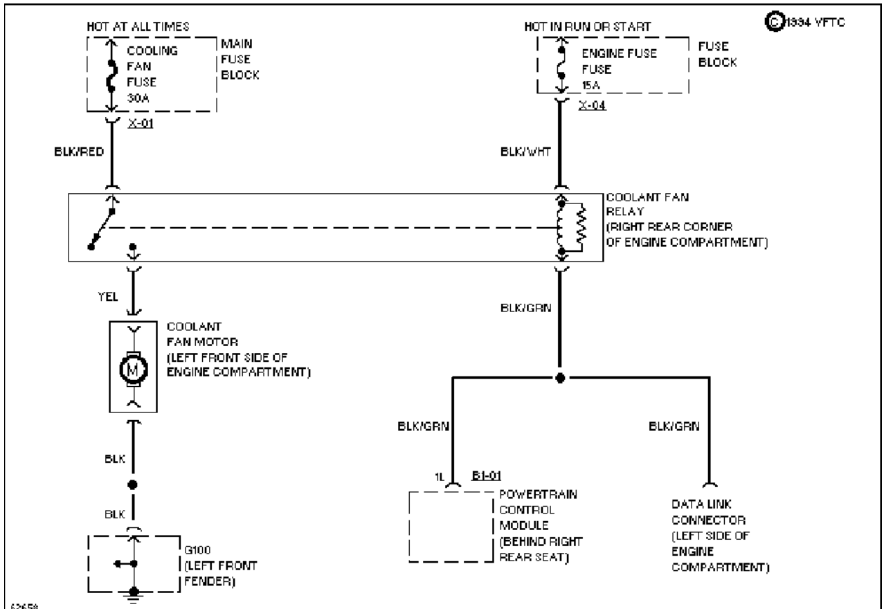
62658 Cooling Fan Circuit
